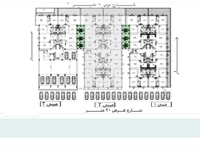
مخططات شقق مبنى 1 - الدور الثاني
